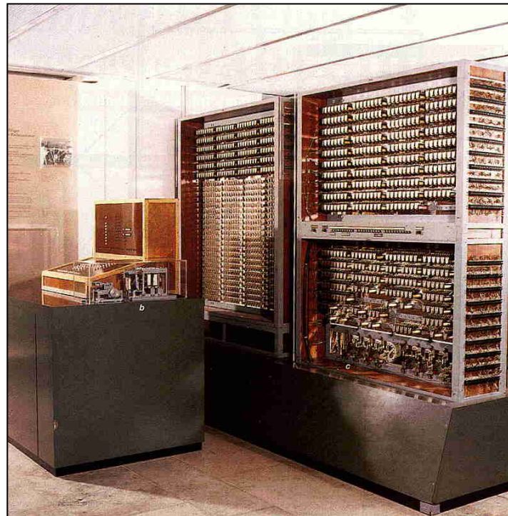
Zuse Z1: 1941
