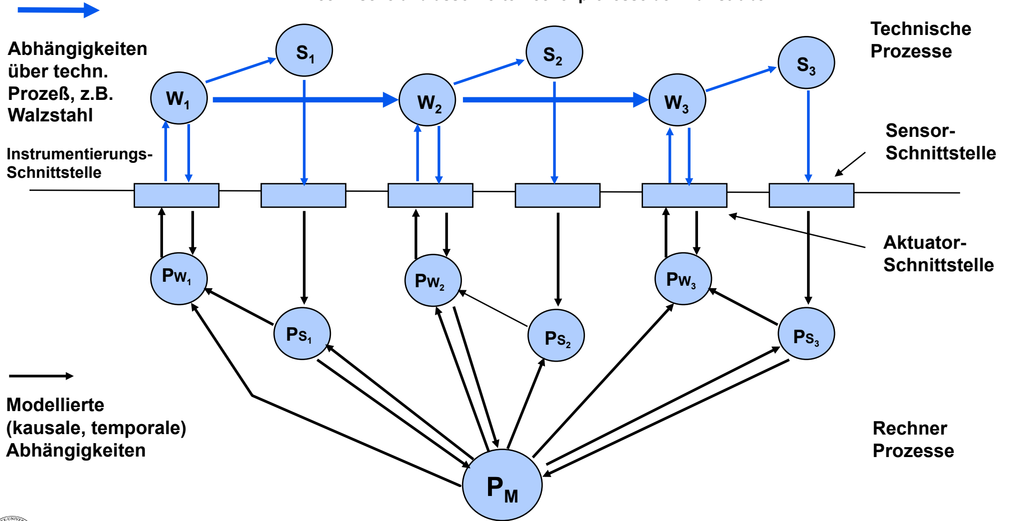
Technische und assoziierte Rechenprozesse der Walzstraße
